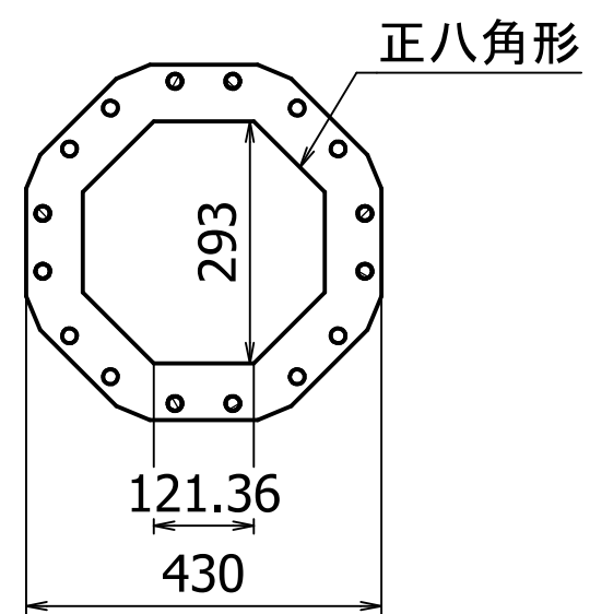
B-B ( 1 : 10 )
